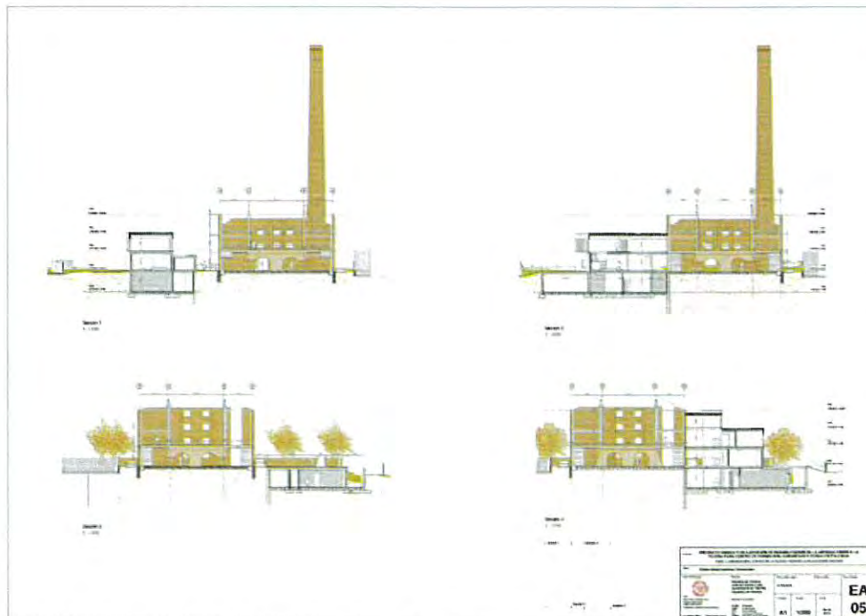
ESTADO ACTUAL. SECCIONES TRANSVERSALES
