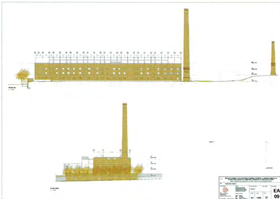
ESTADO ACTUAL. ALZADOS 2.
